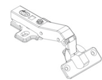
半重疊 ( 三分 ) 安裝
