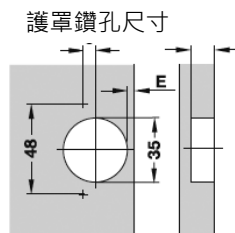
完整重疊 (六分) 安裝
