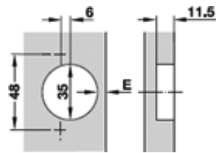
護罩鑽孔尺寸
