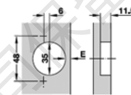
護罩鑽孔尺寸
