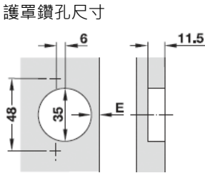
完整重疊 ( 六分 ) 安裝
