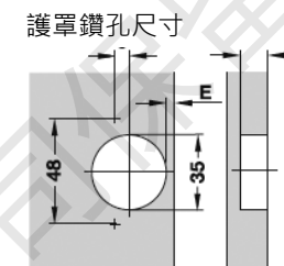
完整重疊 (六分) 安裝
