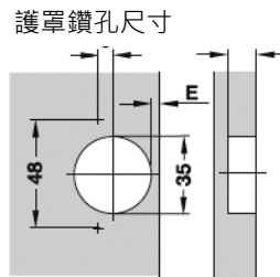
完整重疊 (六分) 安裝
