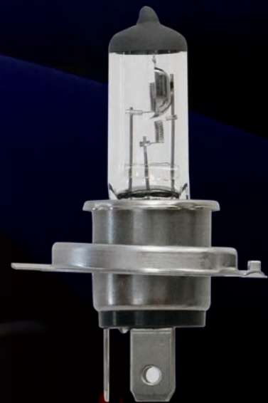
0720 710 1 0720 710 2 大燈 H4(美規9003) 大燈 H4(美規9003) 12V 60/55W 24V 75/70W
