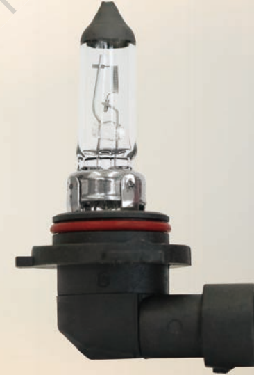
0720 710 4 美規 9006 彎角近燈-HB4 12V 55W
